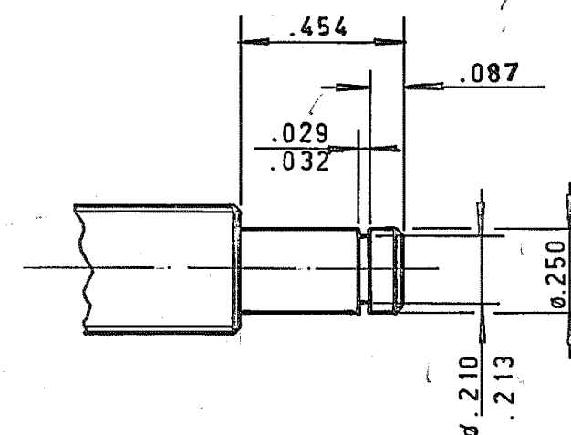
DETALHE W ESCALA - 2:1
